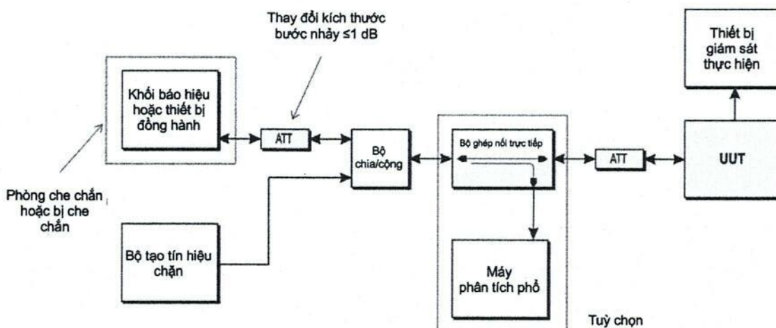
Hình 12 - Cấu hình đo đặc tính chặn máy thu
