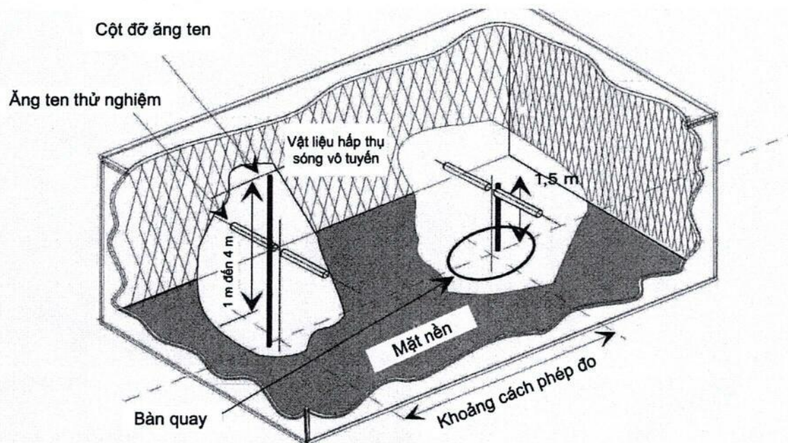
Hình B.2: Phòng bán hấp thụ điện hình
