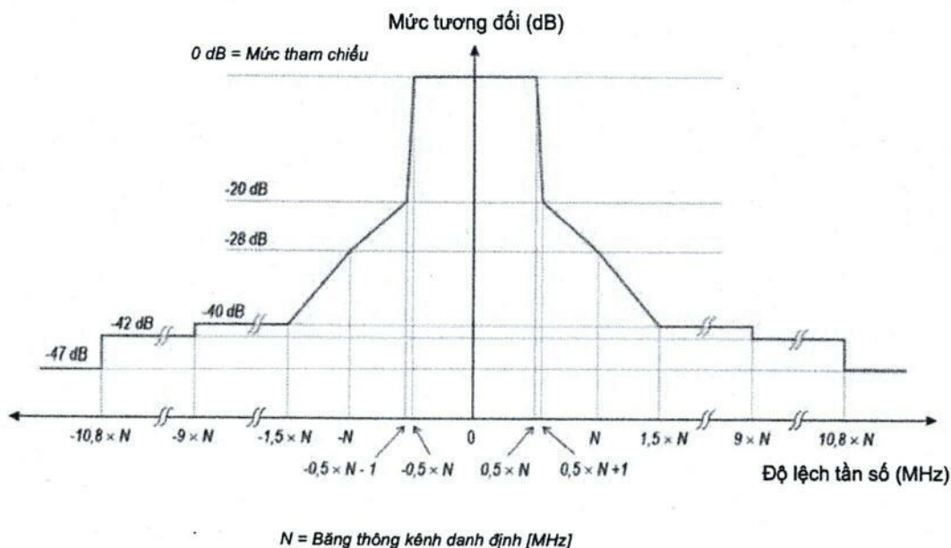
Hình 1 - Mặt nạ công suất phổ phát xạ
