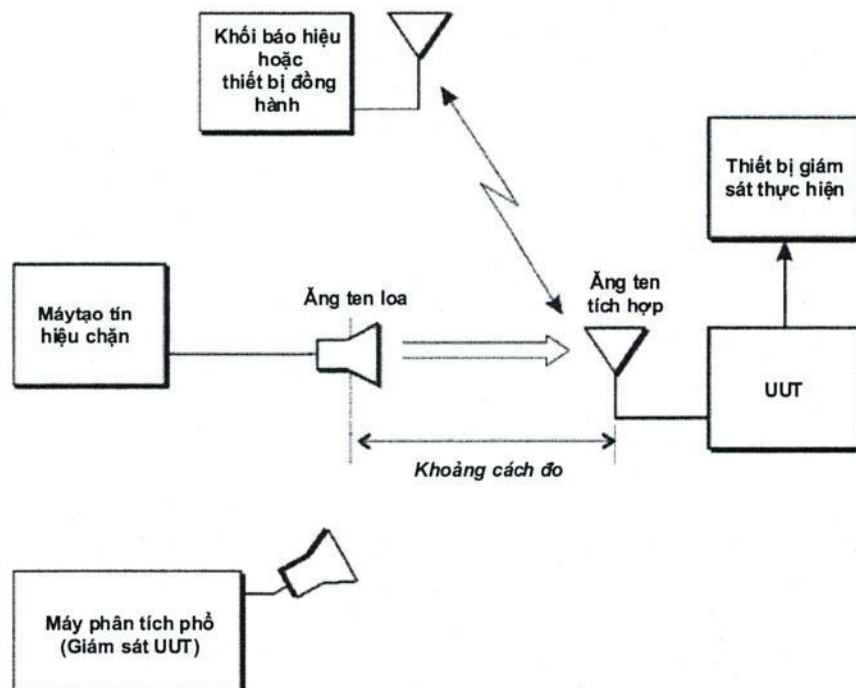
Hình C.4 - Thiết lập phép đo đặc tính chặn máy thu
