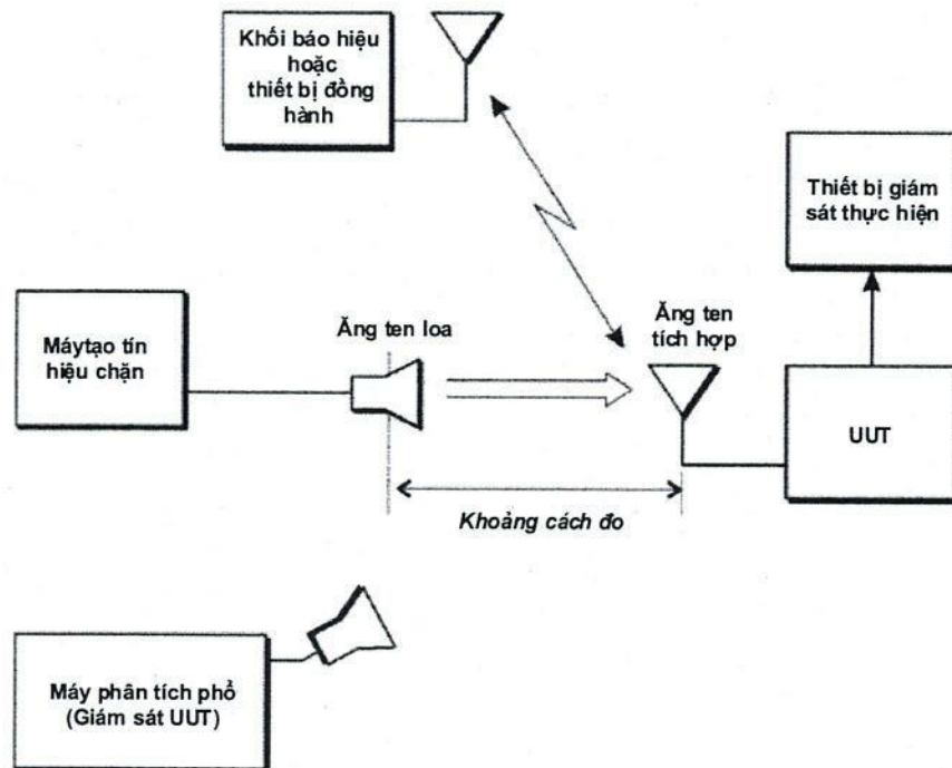
Hình C.6 - Thiết lập phép đo
