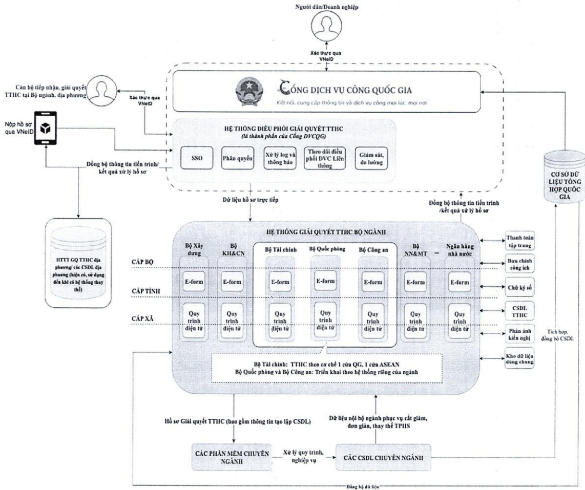
Hình 1: Sơ đồ kiến trúc Hệ thống thông tin giải quyết thủ tục hành chính cấp bộ, cấp tỉnh.
