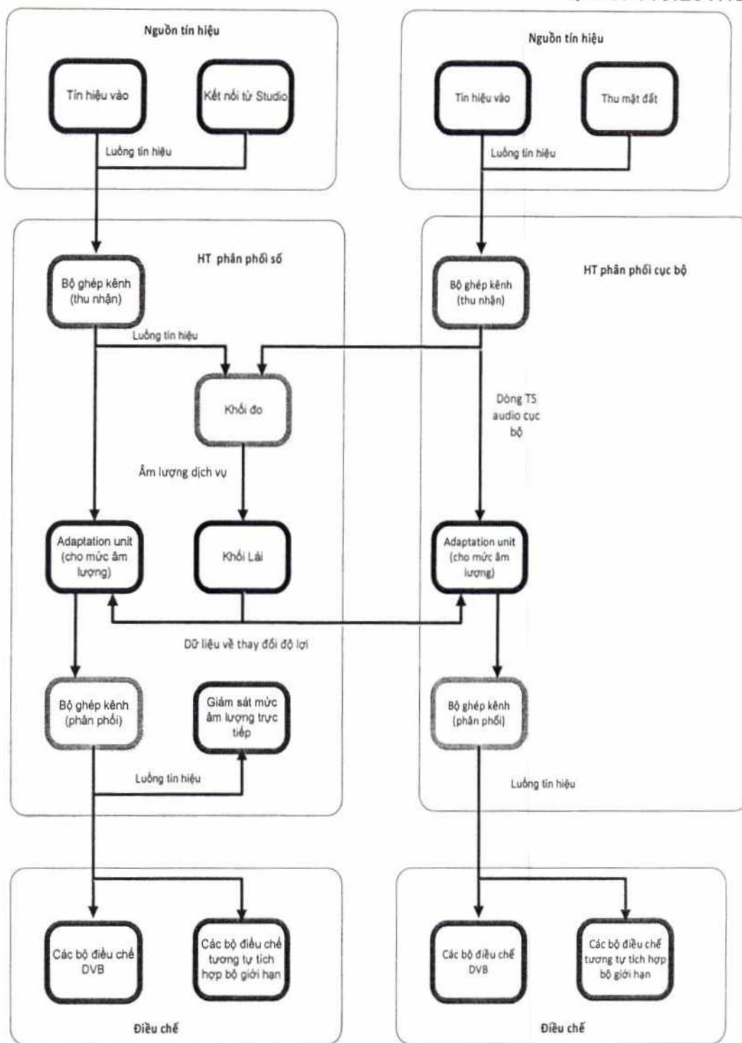
Hình B.4 - Cung cấp và kiểm soát dữ liệu âm lượng từ head-end trung tâm với các head-end cục bộ
