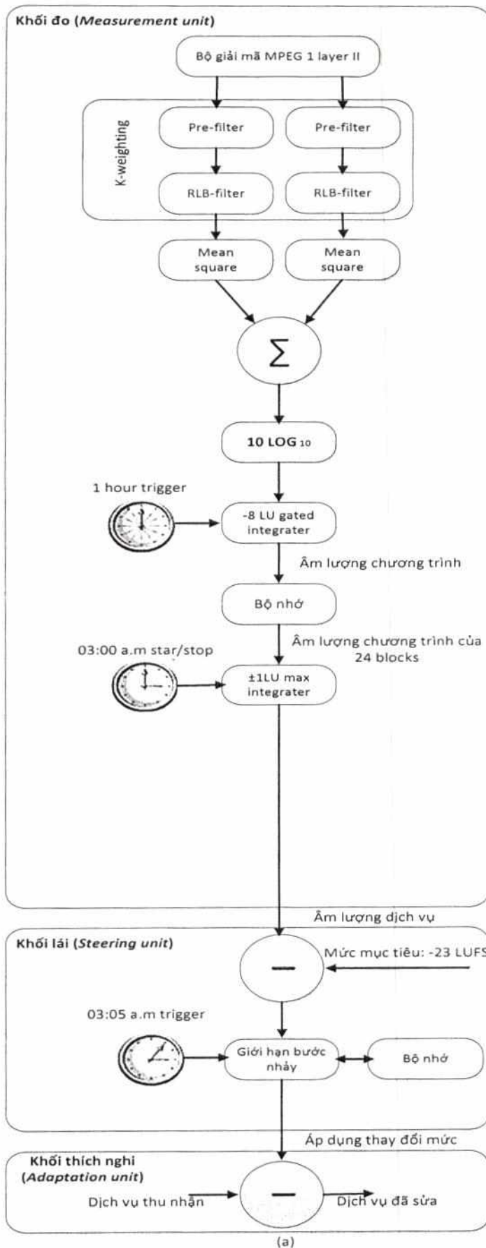
Hình B.2 biểu diễn sơ đồ đo âm lượng và cách thức chuẩn hóa cho các dịch vụ với mã hóa khác nhau.
