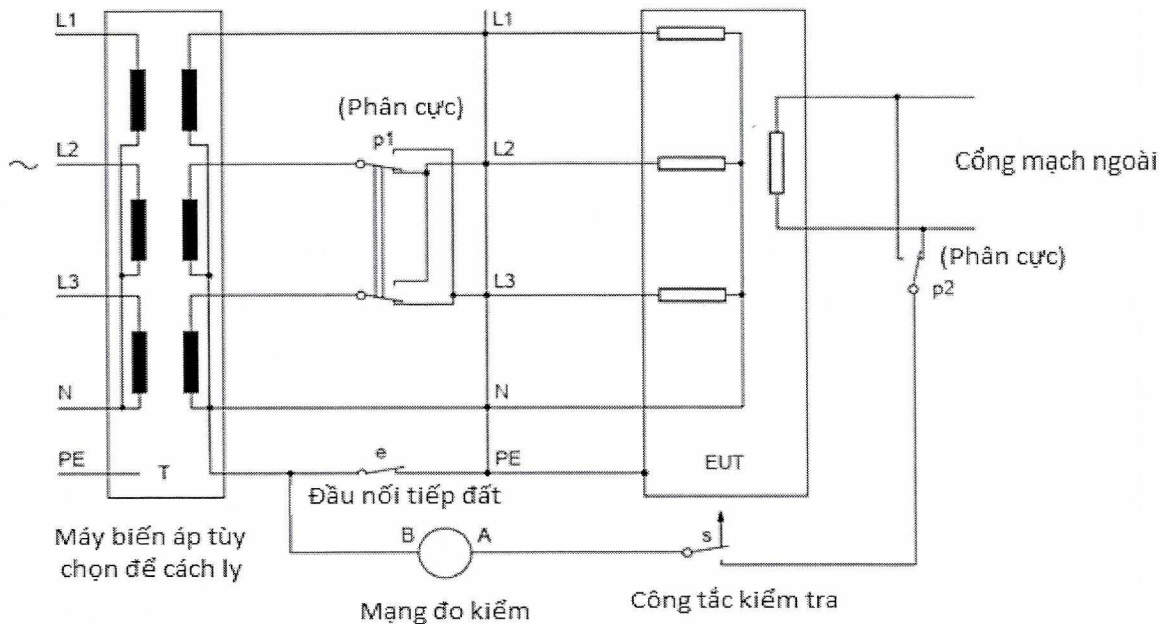
[Hình 33] – Mạch kiểm tra dòng điện tiếp xúc của thiết bị ba pha
